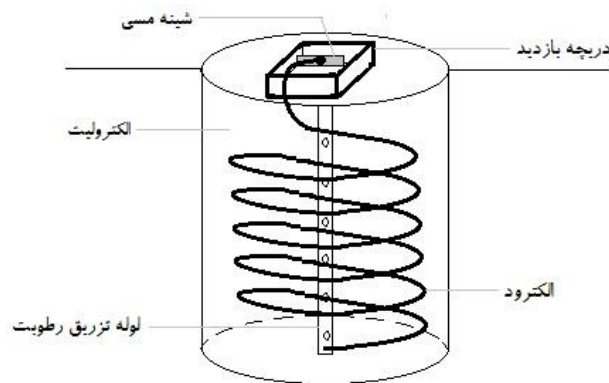
شکل (۵): اجرای الکترود سیمی به صورت فنری با حداقل ۵ دور سیم مسی با مقطع حداقل ۳۵ میلیمترمربع در محیط یک استوانه فرضی به قطر حدود ۵۰ سانتیمتر
